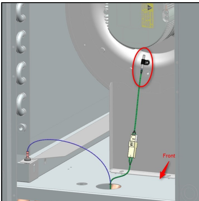
Fig. 3 DAT Sensor Location
